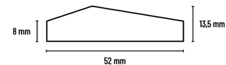
ROOF 1:2
